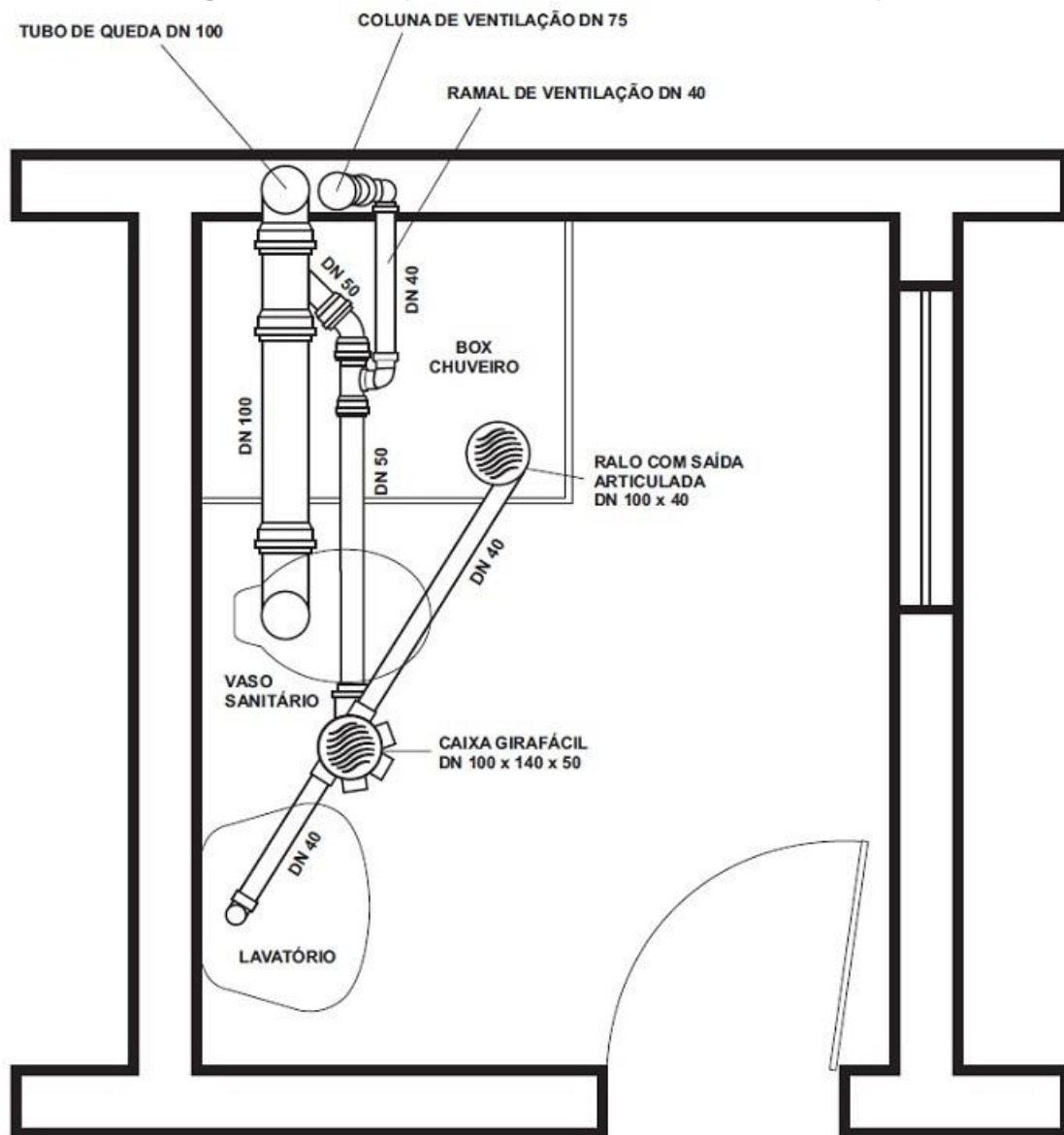
Ligação de Lavatório com Sifão:
